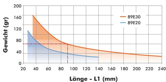
89E20 & 89E30 Gewicht Spannarm
