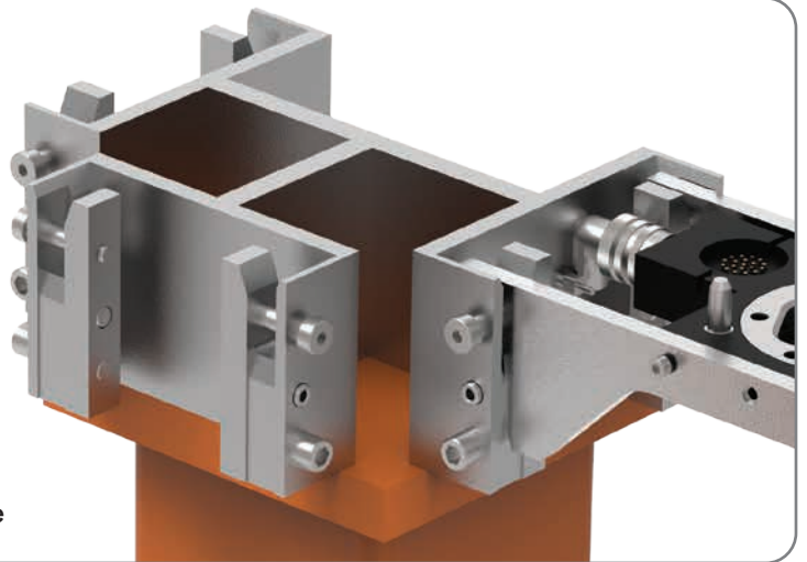
Werkzeugwechsler und Docking-Station der RTP-Serie
