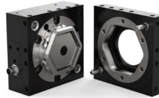
RQC-400 Roboterplatte RTP-400 Werkzeugplatte
