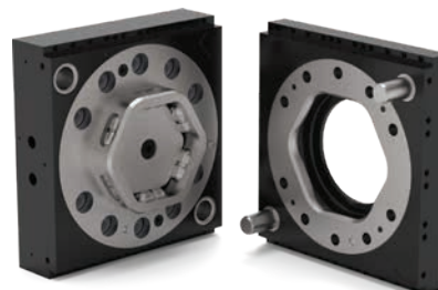
RQC-2400 Roboterplatte RTP-2400 Werkzeugplatte
