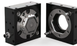
RQC-200 Roboterplatte RTP-200 Werkzeugplatte
