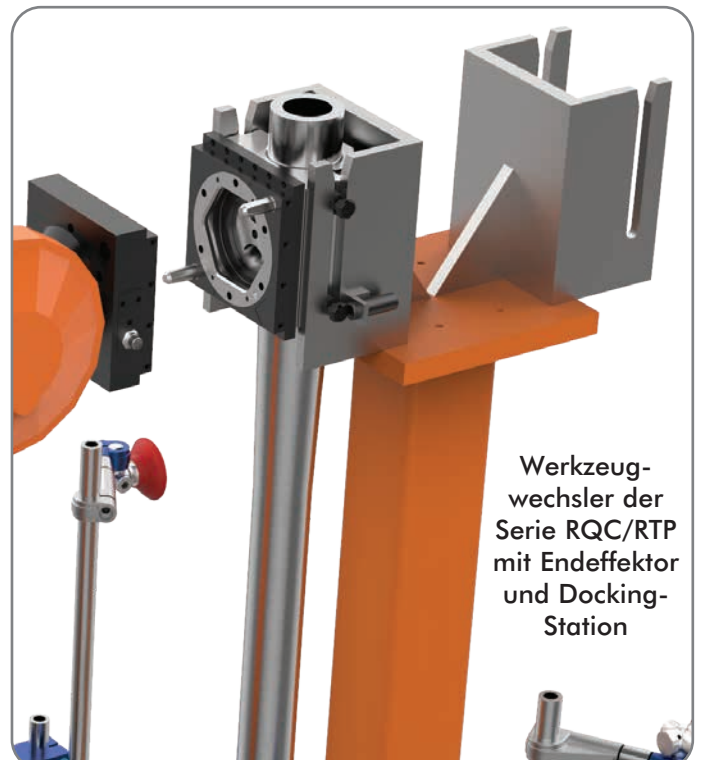
Werkzeugwechsler und Docking-Station der TP-Serie
