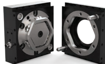
RQC-1200 Roboterplatte RTP-1200 Werkzeugplatte
