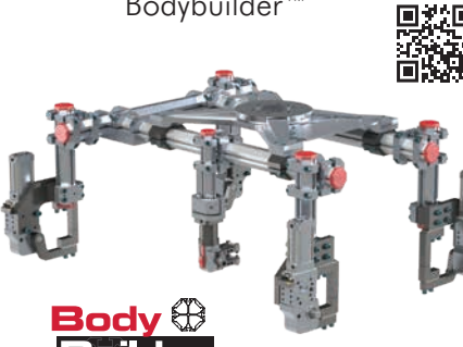
Préhenseurs octogonaux Bodybuilder™
