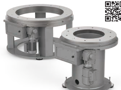
Indexeur Ring Drive
