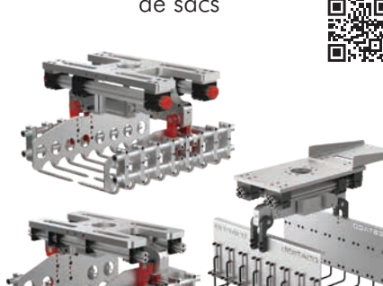
Préhenseur de palettisation de sacs
