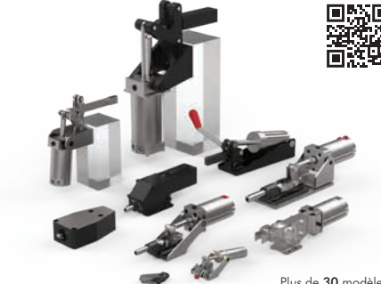
Serrage pneumatique à trois points
