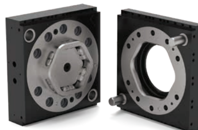
RQC-2400 Roboterplatte RTP-2400 Werkzeugplatte
