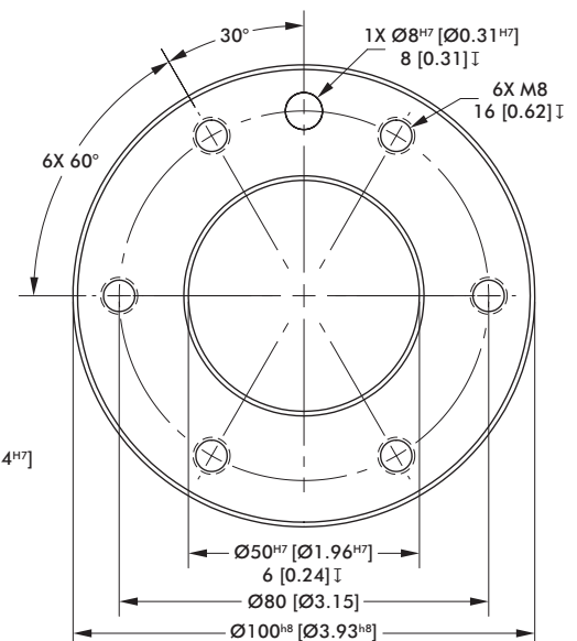
ISO-9409-1-80-6-M8
