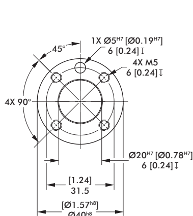
ISO-9409-1-31.5-4-M5
