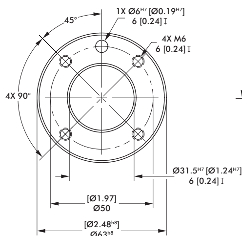
ISO-9409-1-50-4-M6
