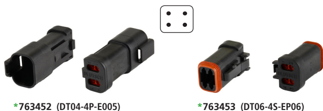
*763452 (DT04-4P-E005)
