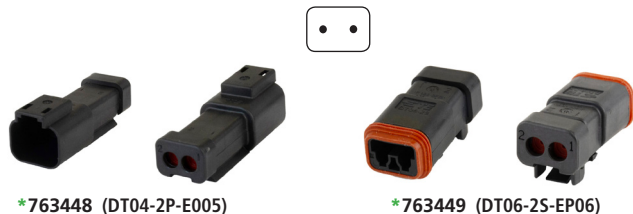
*763448 (DT04-2P-E005)
