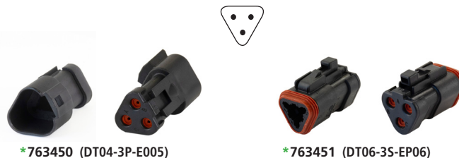
*763450 (DT04-3P-E005)
