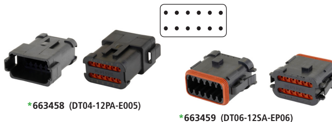
*663459 (DT06-12SA-EP06)
