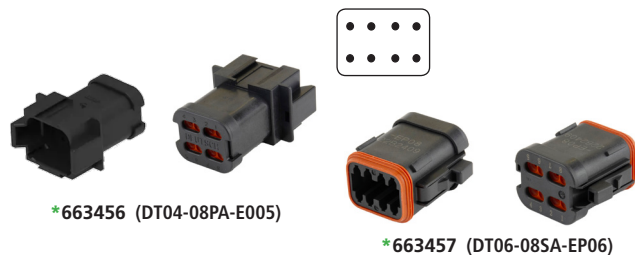
*663457 (DT06-08SA-EP06)
