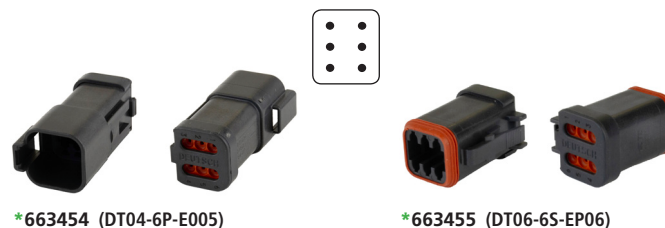
*663454 (DT04-6P-E005)
