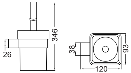
CELIA TOILET BRUSH HOLDER NR4688CH/NR4688MB/NR4688BN
