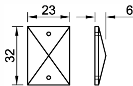
B R20015-032-00-01 W23*L32*T6mm
