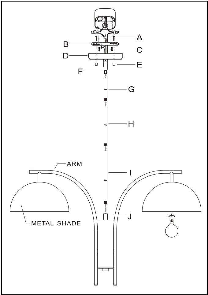
ITEM NO: 513771; 513772
