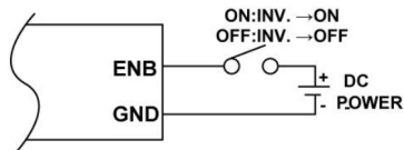
Wiring Options
