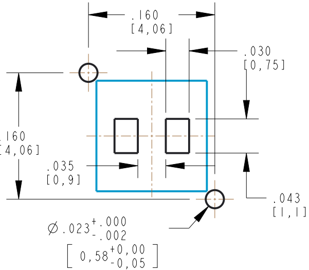
SINGLE COLOR MINI PLCC-2 598-8CX0-107F LAYOUT
