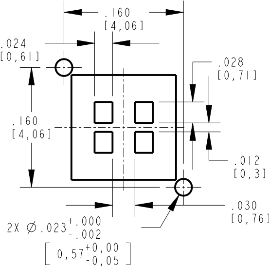
BI-COLOR 0606 598-84X0-207CF LAYOUT
