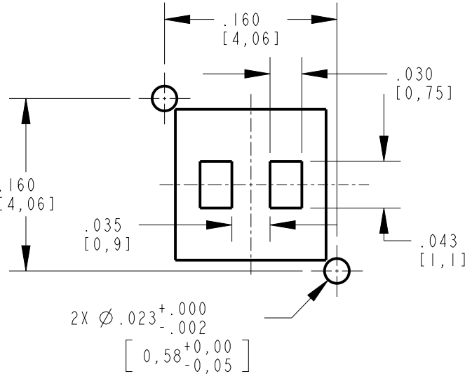
SINGLE COLOR MINI PLCC-2 598-8CX0-107F LAYOUT
