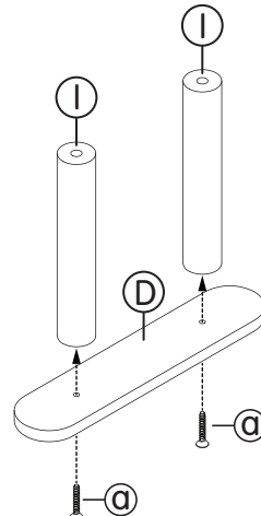
Detail : D
