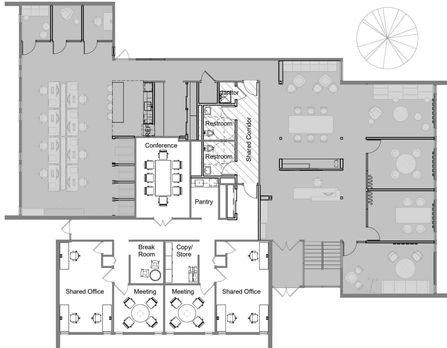
1 Tenant Plan 3/32" = 1'-0"
