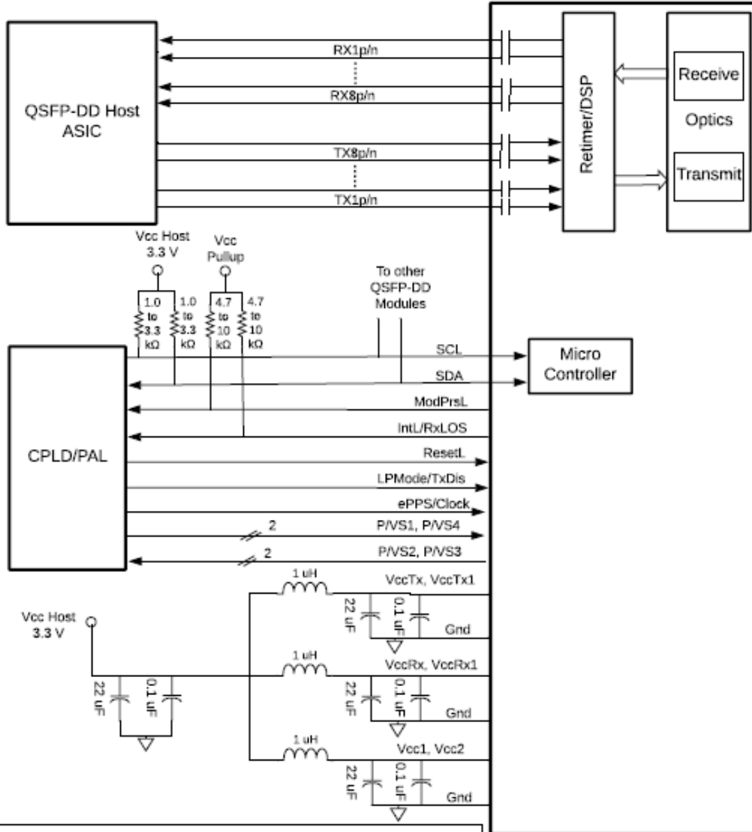
QSFDD/QSFDD800 Optical Module
