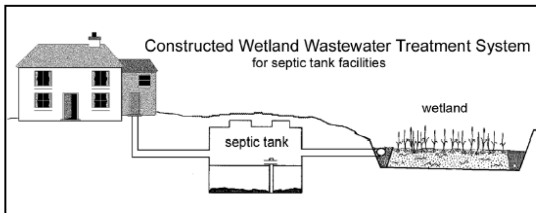
obr. Systém umělého mokřadu u domu se septikem
