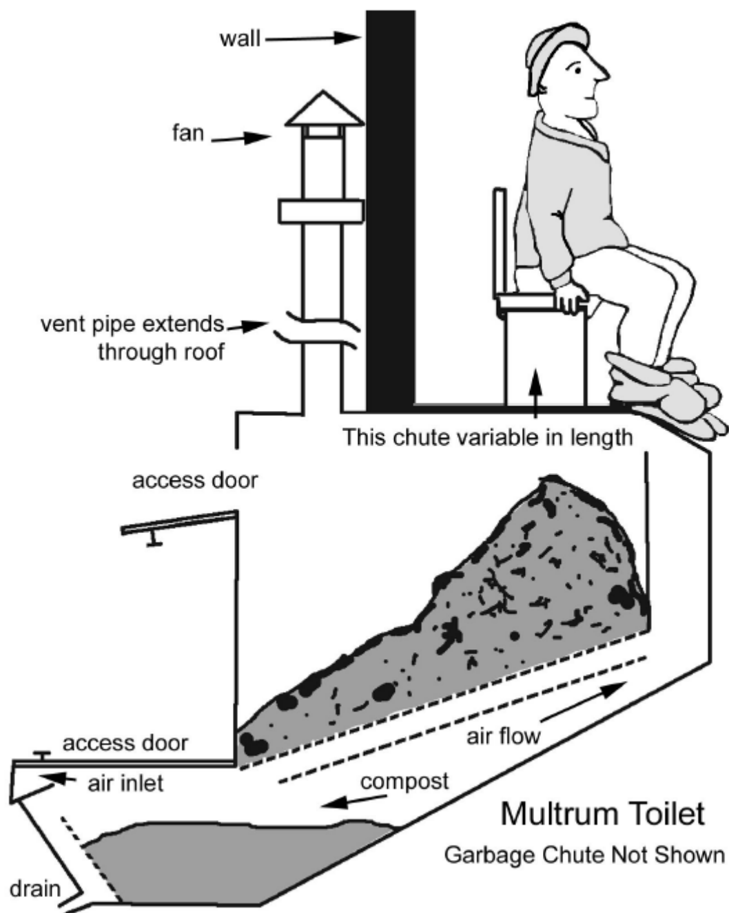
obr. Toaleta Multrum
