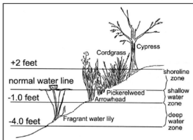
obr. 9.7 Vodní rostliny v pobřežní zóně, zóně mělké vody a hluboké vody; shora cypřiš, tráva spartina, slanorožec, šípka, leknín
