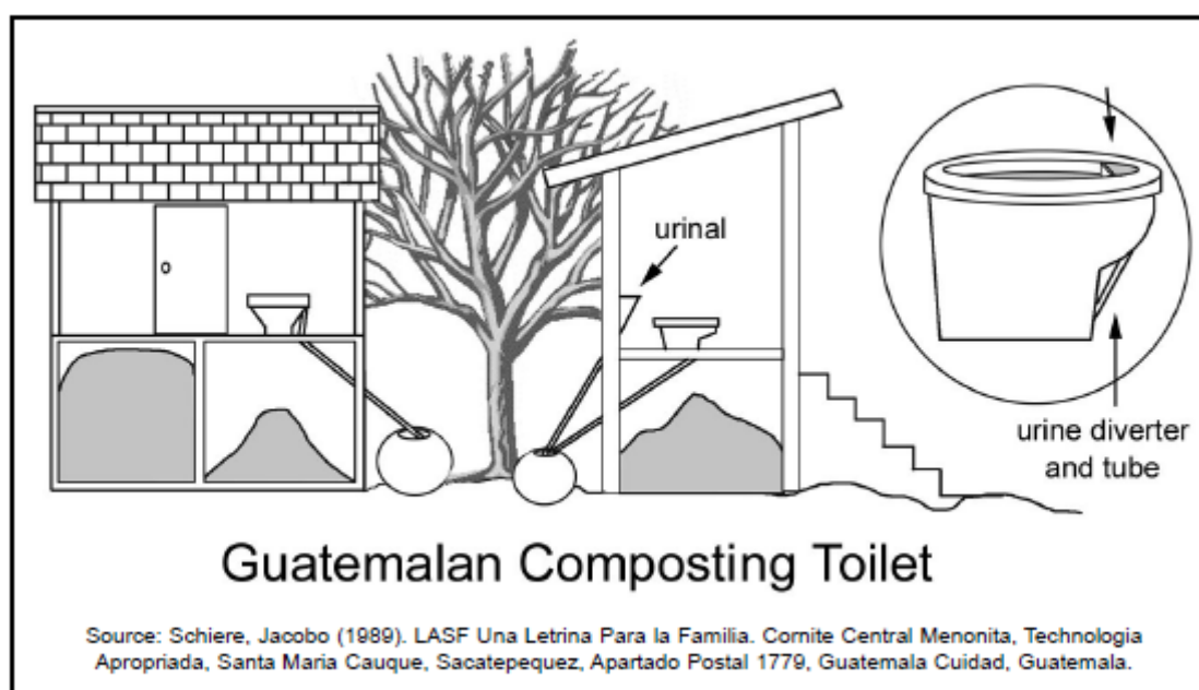
obr. Guatemalská kompostovací toaleta se separací moči
