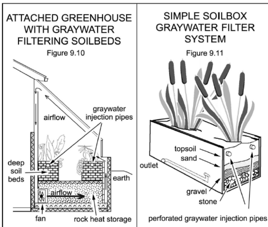
obr. 9.10 Ke stěně domu je zvenku přistavěný skleník se záhony na čištění šedé vody. Pod úroveň venkovní půdy je v podlaze skleníku vrstva štěrku na akumulaci tepla. Vespod umístěný ventilátor zajišťuje cirkulaci vzduchu. V hlubokých záhonech s půdou jsou rostliny zavlažované šedou vodou čerpanou z domu.
