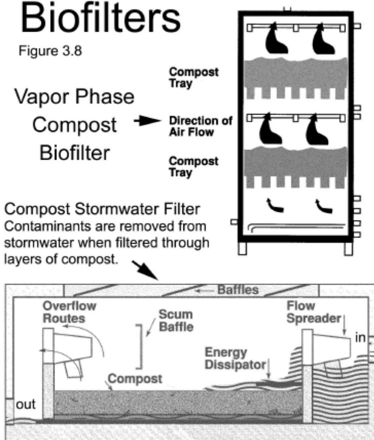
obr. 3.8 Biofiltry na vzduch a na vodu z přívalemých srážek
