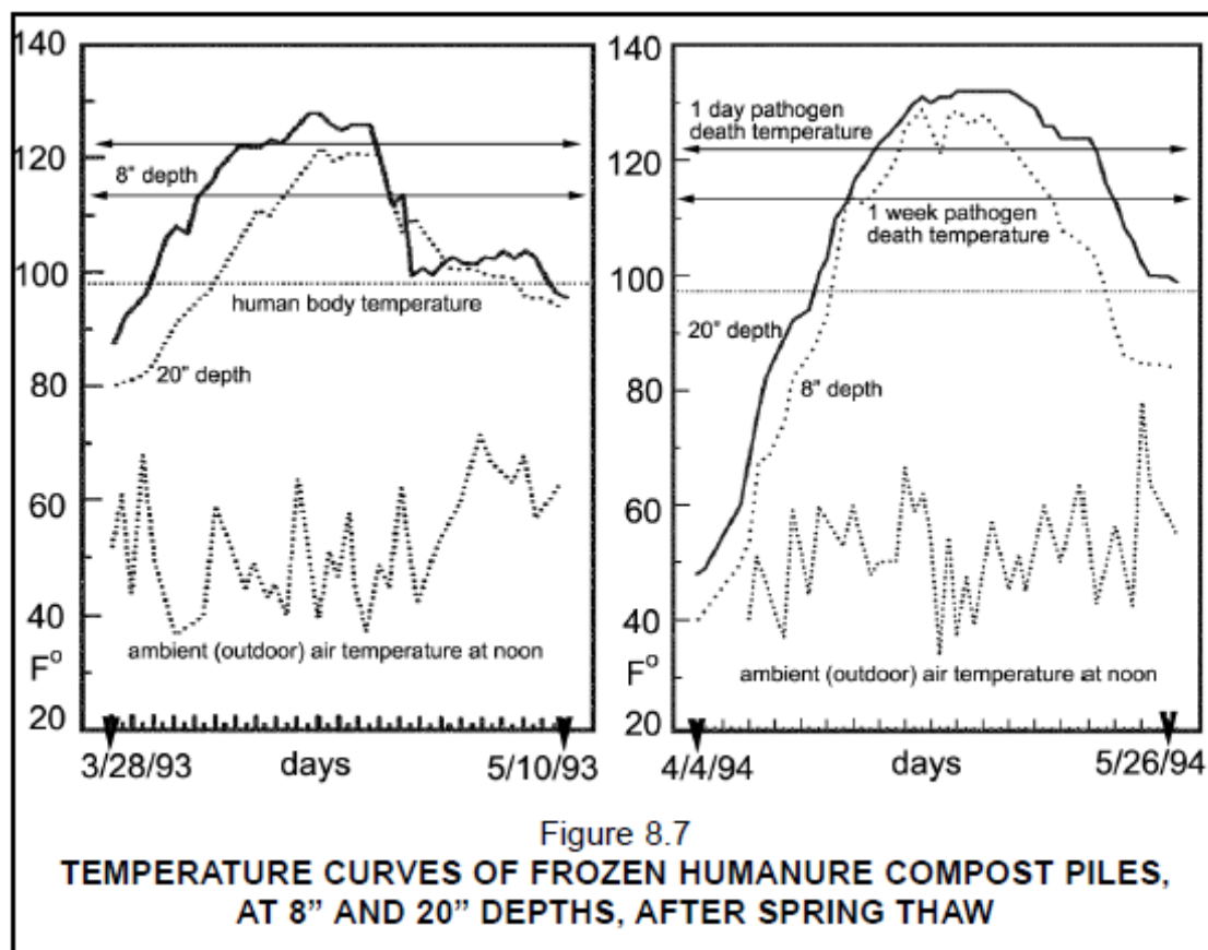
obr. 8.7 Vývoj teploty v hromadách kompostu při jarním tání ve dvou různých hloubkách
