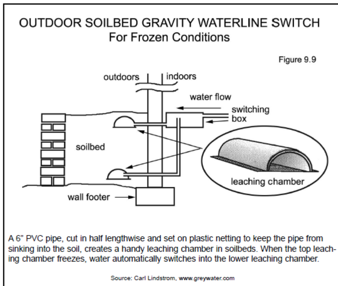
obr. 9.9 Venkovní zasakovací záhon na vodu, která vytéká gravitací z čističky umístěné v domě (vpravo) je určen pro oblasti, kde v zimě mrzne. Kus podélně rozříznuté trubky o průměru 6 palců chrání vyústění potrubí vedoucího z domu do záhonu ve dvou různých hloubkách v půdě. Potrubí je podloženo plastovou sítí, aby v půdě nepropadalo. Když půda kolem mělčeji umístěné trubky zamrzne, voda bude vytékat z druhé, hlouběji zakopané, a dál se vsakovat.
