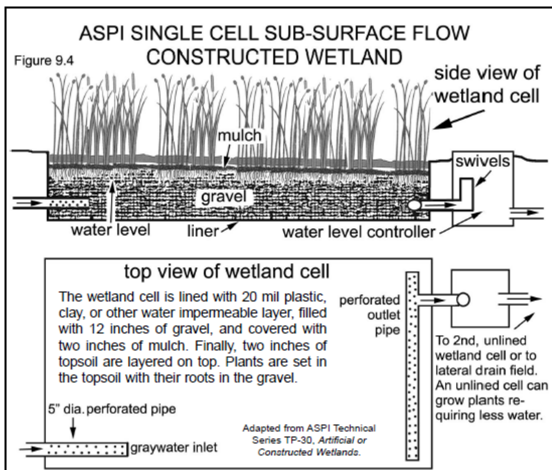
obr. 9.4 Jednkomorová průtoková podpovrchová kořenová čistička (umělý mokřad) je vyložená plastovou fólií, jilem nebo jiným nepropustným materiálem, naplněná 12 palci šterku a pokrytá 2 palci mulče. Na povrchu mohou být dva palce zeminy, do níž jsou
