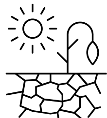
El Niño
