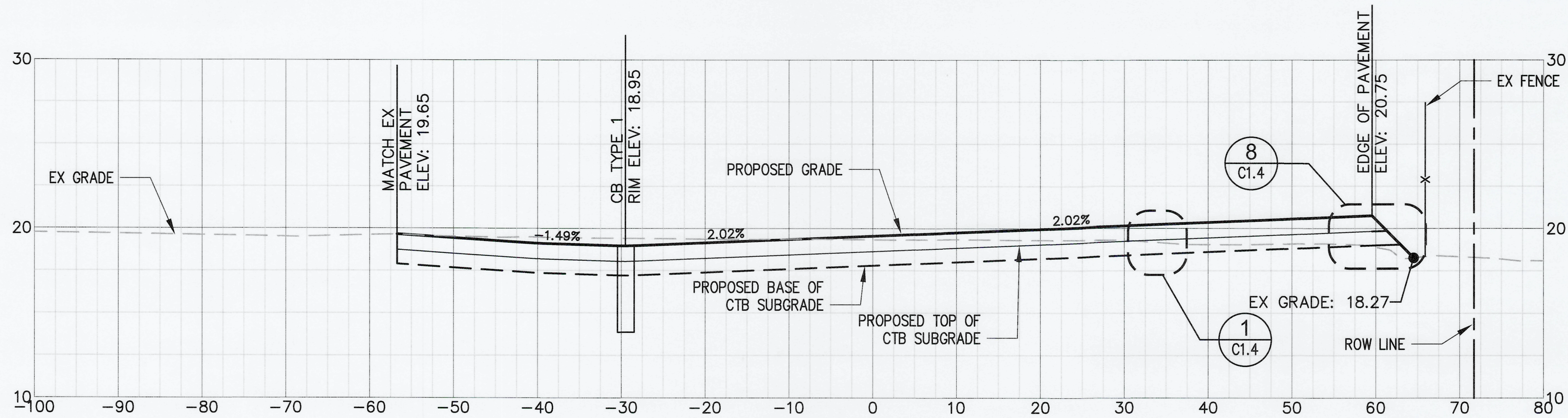
B SITE SECTION SCALE: HORZ 1:10, VERT 1:5
