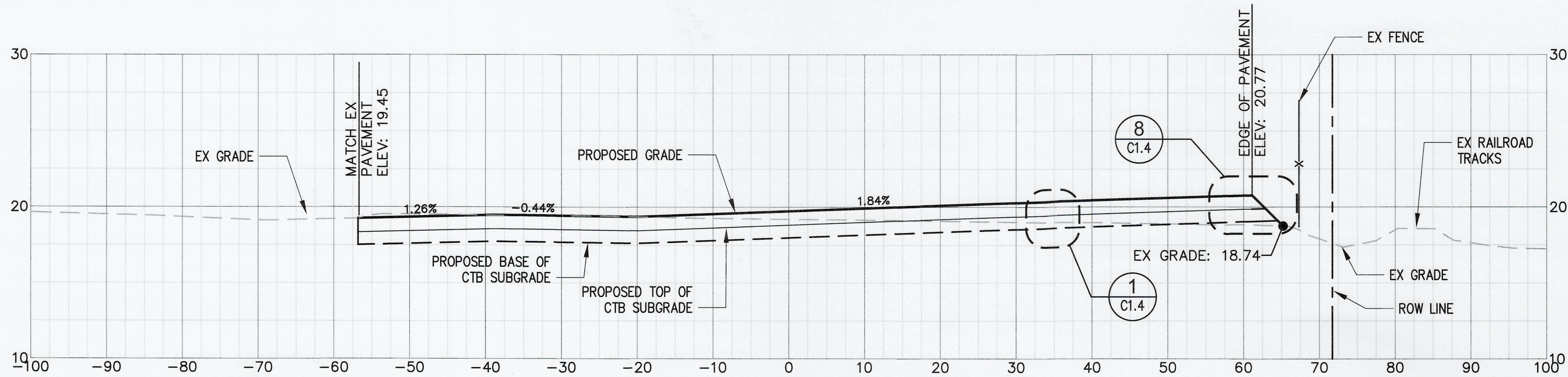
A SITE SECTION SCALE: HORZ 1:10, VERT 1:5
