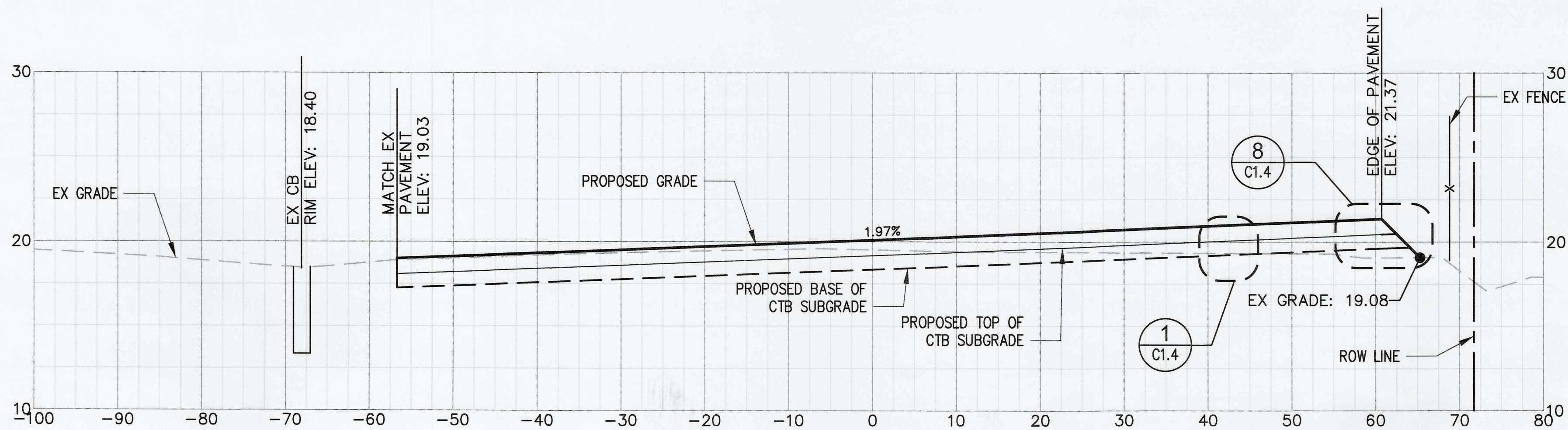
C SITE SECTION SCALE: HORZ 1:10, VERT 1:5
